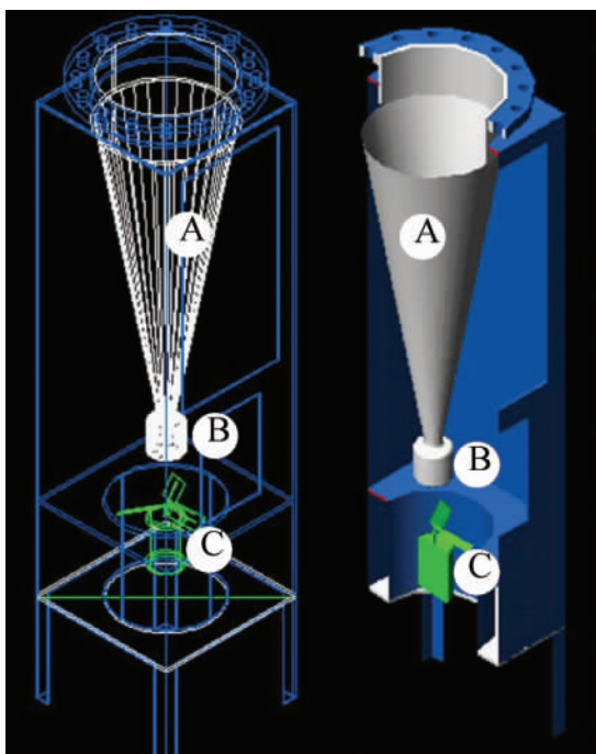
图2 科云 ST-1B 型吸虫塔机箱内部结构示意图
