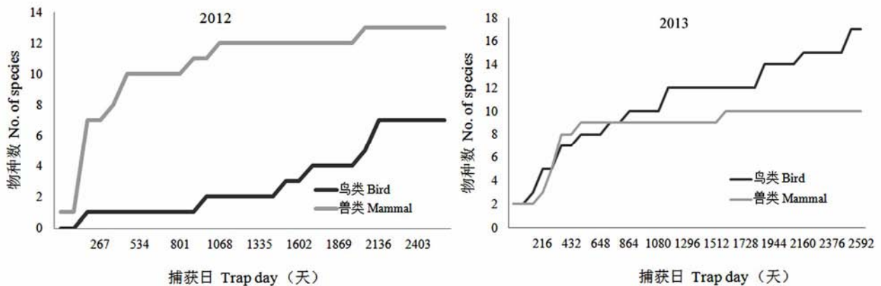
图2 西双版纳森林动态监测样地及周边区域红外相机拍摄鸟类与兽类累计曲线
